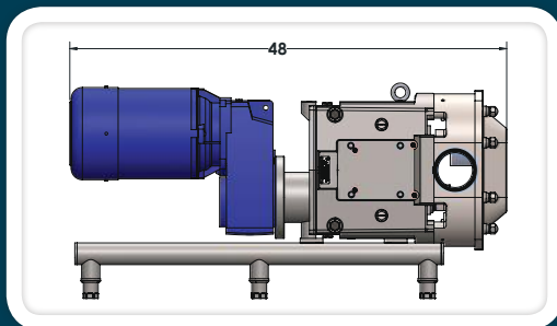
ZP-CC Dimension
