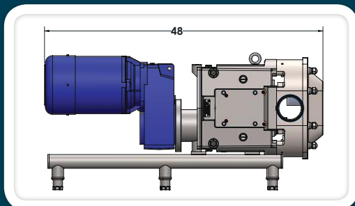
ZP-CC Dimension
